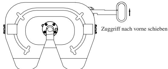
Abbildung 10 - Öffnen der Sattelkupplung
