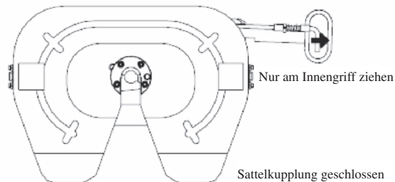
Abbildung 9 - Öffnen einer Sattelkupplung mit Interlock-Zuggriff
