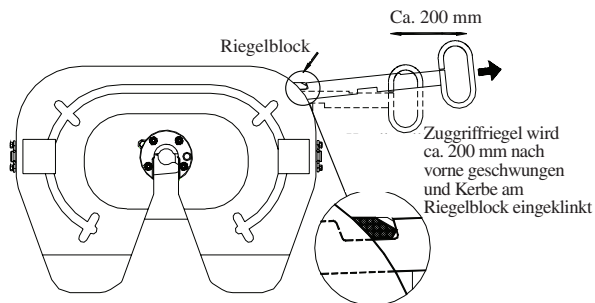
Abbildung 3 - Sattelkupplung in geöffneter Position
